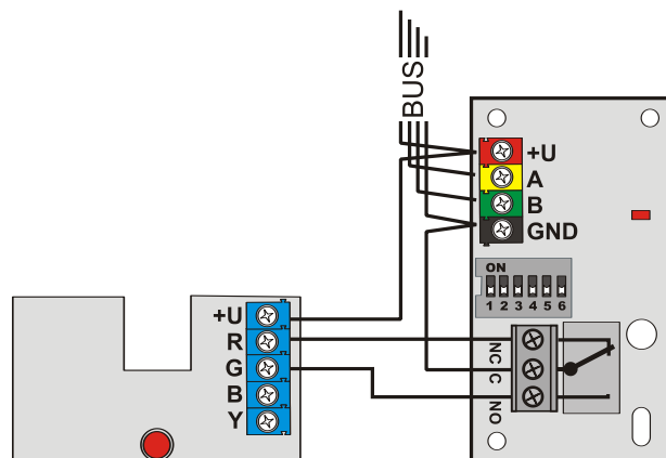
Figura: exemplu de conexiune ce permite semnalizarea bicoloră a stării unui modul de ieșire
