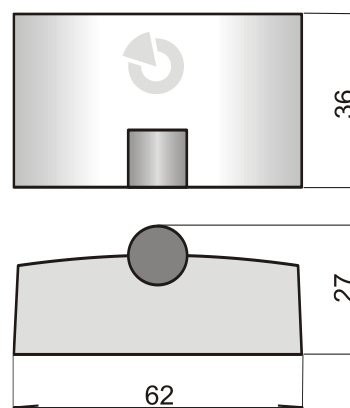
Figura: dimensiunile indicatorului JA-111I .
