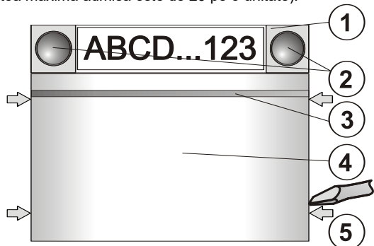
Figura: 1 – segment de control ; 2 – butoane segment ; 3 – buton de activare a iluminatului 4 – modul RFID ; 5 – declanșatoare ale butoanelor de apăsare pentru deschiderea modulului
