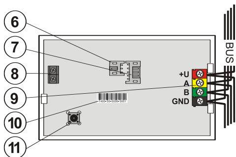
Figura 6 – conector modul audio ; 7 – conector al segmentului de control ; 8 – terminal pentru conectarea modulului audio la panoul de control , 9 – terminale bus , 10 – cod de producție ; 11 – contact tamper
